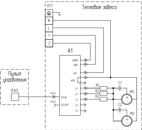
Схема электрическая принципиальная воздушной завесы ВНС-Н20А-PS:
