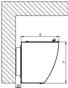
Расположение кронштейнов для горизонтального установки
