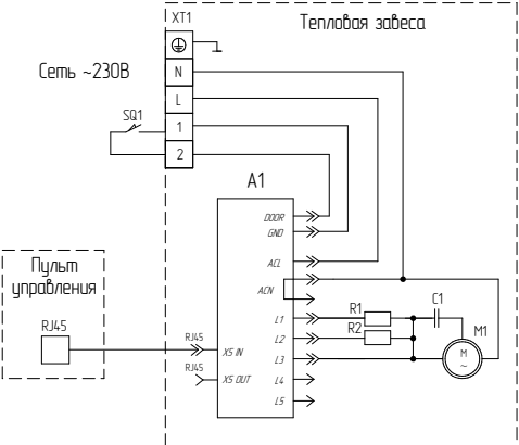
Схема электрическая принципиальная воздушной завесы ВНС-Н15А-PS:
