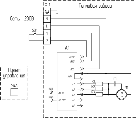
Схема электрическая принципиальная воздушной завесы ВНС-Н10А-PS:
