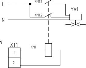
Контроллер BRC-W
