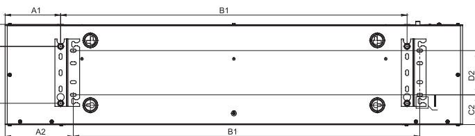
Расположение кронштейнов для установки завесы на шпильки
